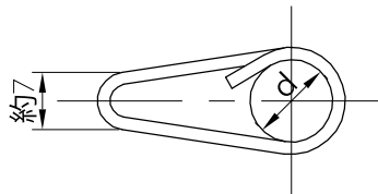
L型サポートステンレスバネの寸法
